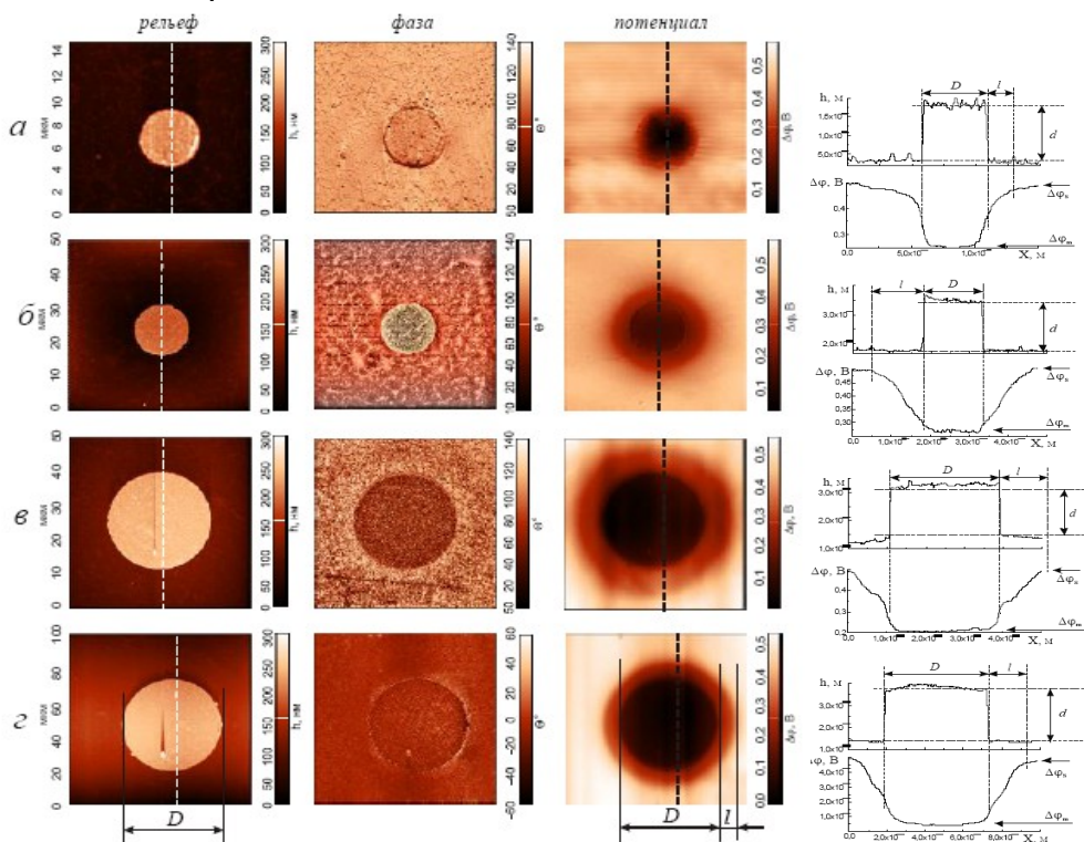
Рис. 2. Двумерные АСМ изображения рельефа, фазового контраста, КРП, пространственных h(x) и потенциальных \Delta\varphi(x) сечений рельефов поверхности nGaAs(100) с концентрацией доноров 3 \cdot 10^{15} \text{ cm}^{-3} с расположенными на ней металлом (Au) толщиной d \approx 0,2 \text{ мкм} с диаметрами D: а) 5 мкм; б) 15 мкм; в) 30 мкм и г) 50 мкм.
